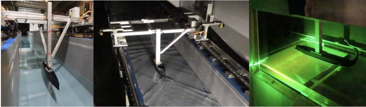
Figure 2 : ( gauche ) bassin d'essais des carènes de l'Institut Pprime avec son chariot de traction et une maquette de bateau maritime ; (milieu) sillage transcritique d'un bateau fluvial avec émission de solitons (droite) vélocimétrie par image de particules de l'écoulement autour d'une galère antique.
