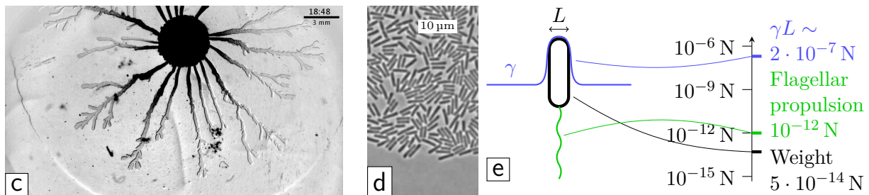
(c) Étalement dendritique de bactéries à partir de la colonie mère au centre. Le mouvement est confiné à la surface d'un gel nutritif, vu ici de face. (d) Avant d'un dendrite à fort grossissement. Une frontière très nette délimite la population dense de bactéries. (e) Les forces capillaires dominant de plusieurs ordres de grandeur les forces que les bactéries parviennent à générer à l'aide des flagelles.
