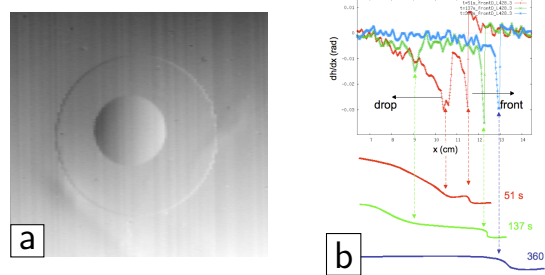
(a) Mesure de la pente dans la direction gauche-droite d'une goutte de surfactant, qui montre un front de gonflement qui s'éloigne de la goutte. (b) Le profil radial du front reste invariant au cours du temps.
